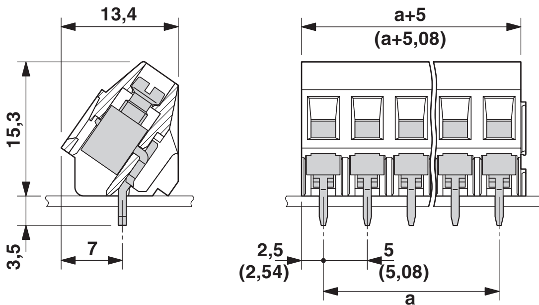
Rysunek wymiarowy
