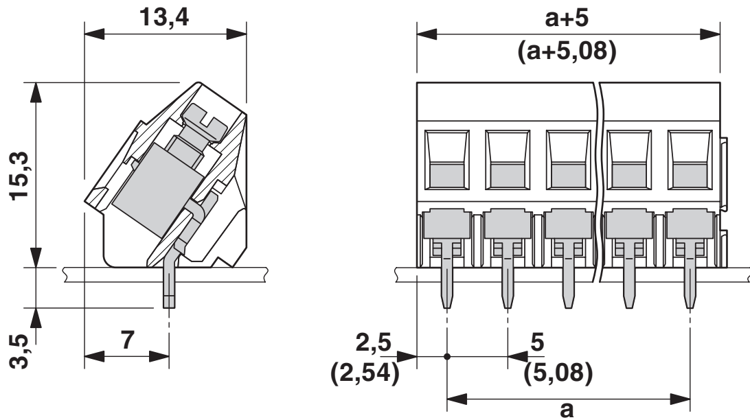
Rysunek wymiarowy
