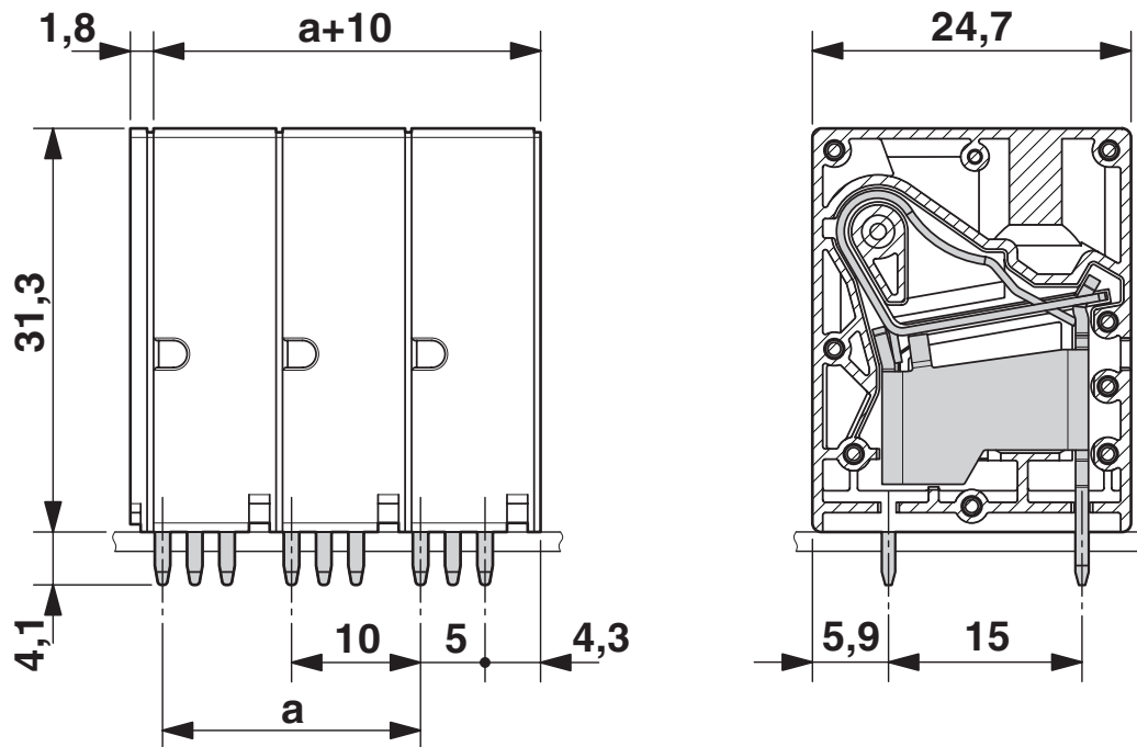
Rysunek wymiarowy
