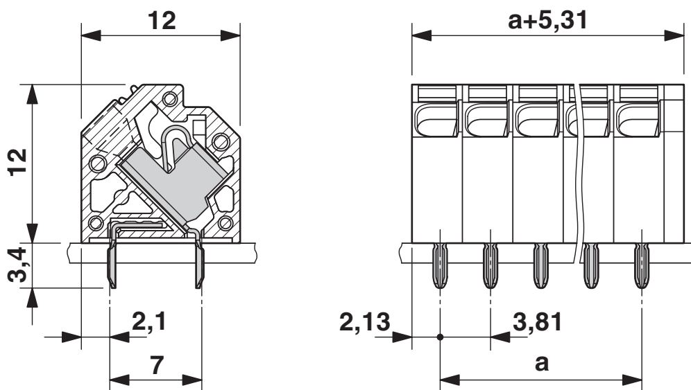
Rysunek wymiarowy
