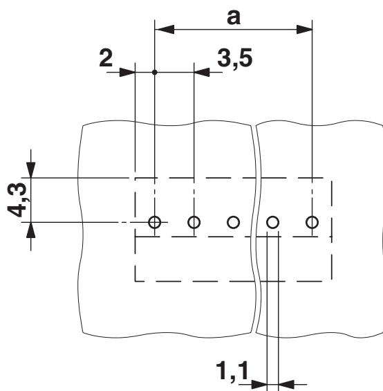
Rysunek wymiarowy
