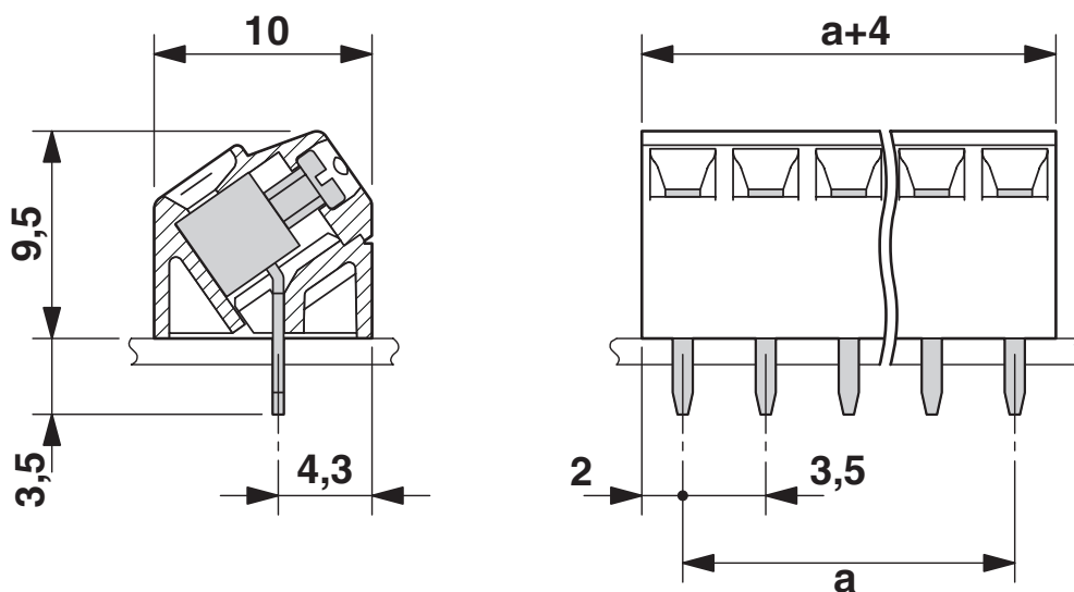
Rysunek wymiarowy
