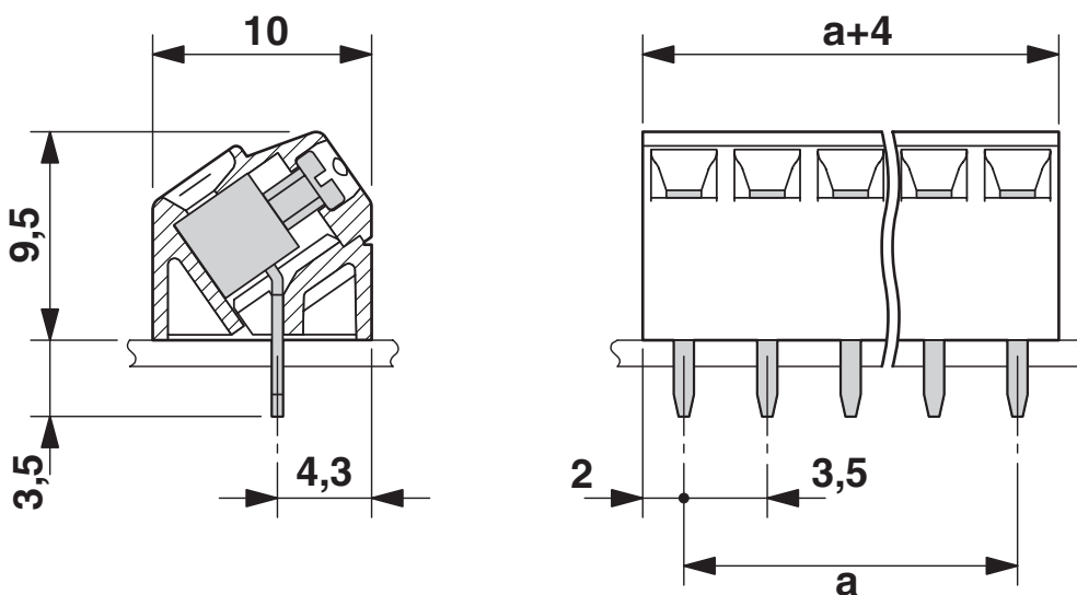
Rysunek wymiarowy
