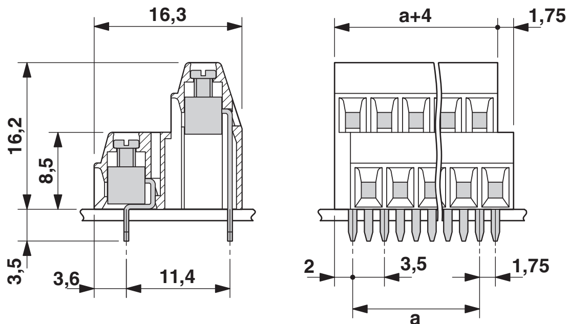
Rysunek wymiarowy
