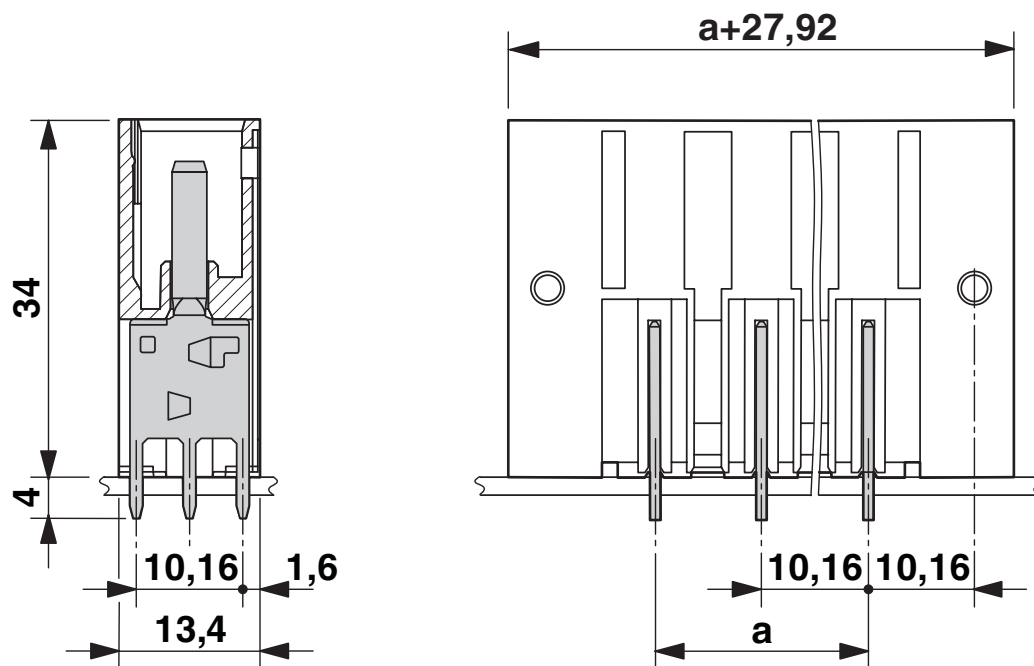
Rysunek wymiarowy
