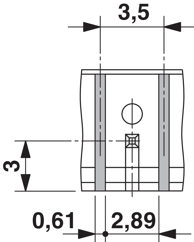
Rysunek wymiarowy
