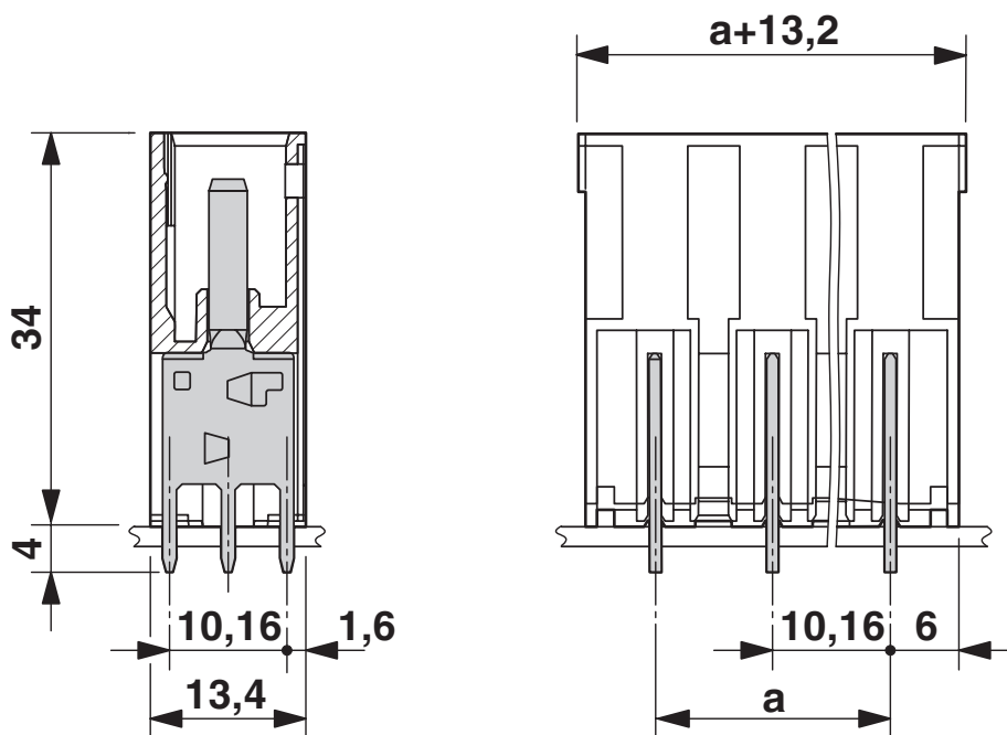
Rysunek wymiarowy
