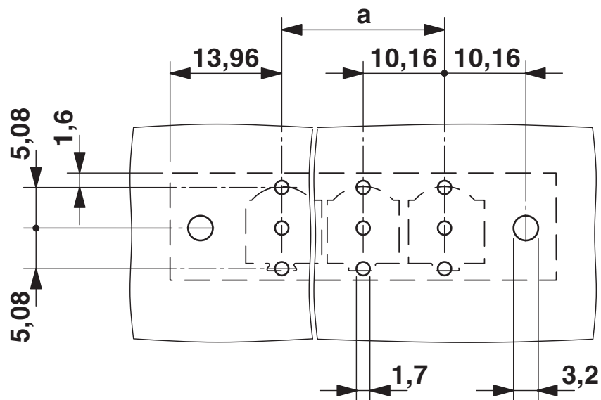
Otworowanie/geometria płytek lutowiczych
