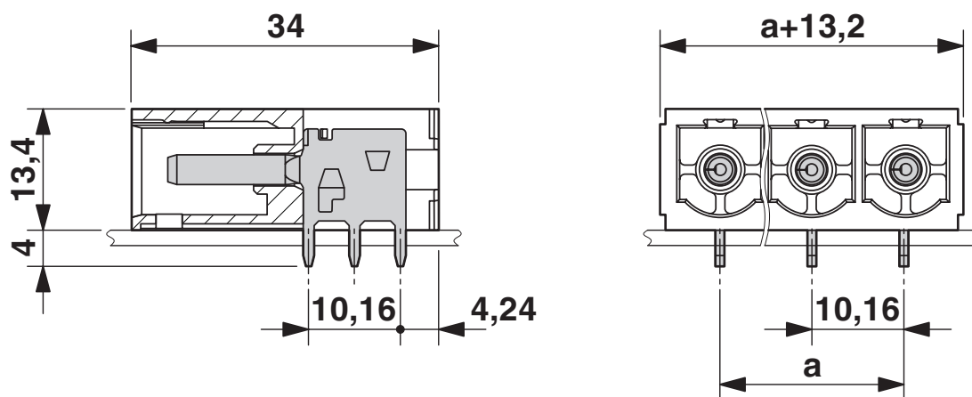
Rysunek wymiarowy
