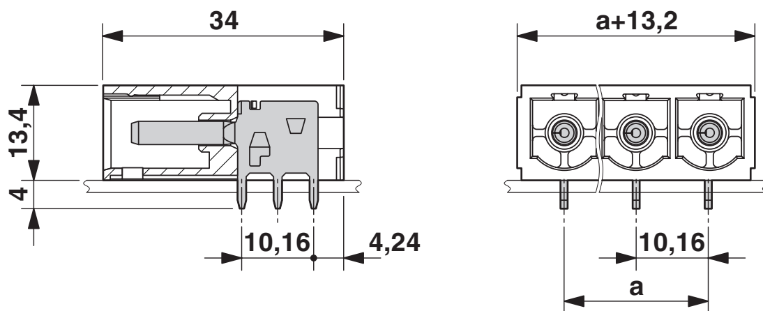
Rysunek wymiarowy
