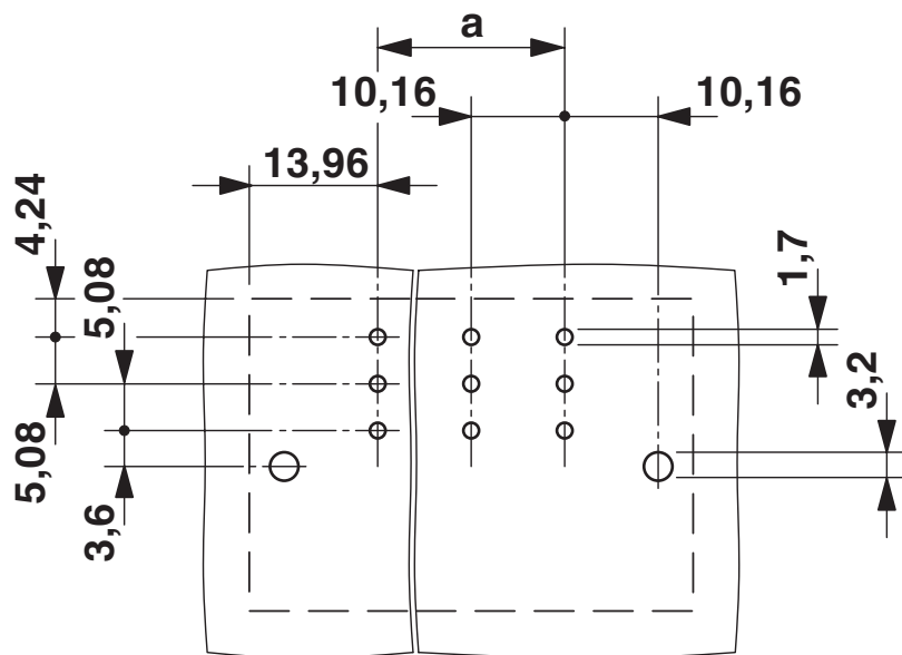
Otworowanie/geometria płytek lutowiczych
