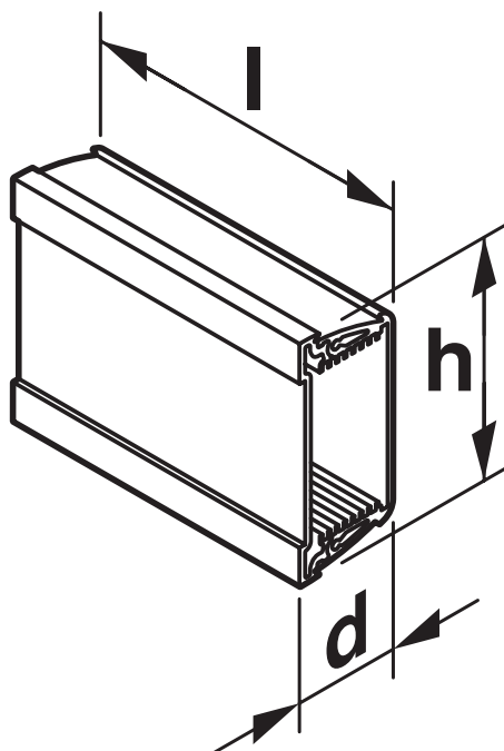
Rysunek wymiarowy
