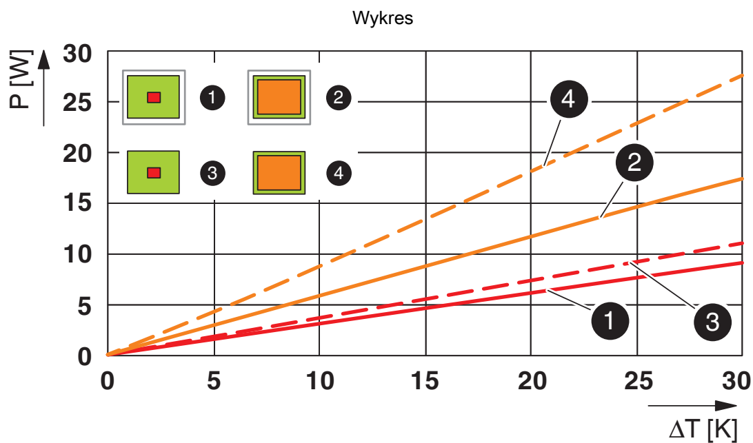
Wykres strat mocy 0 K ... 100 K
