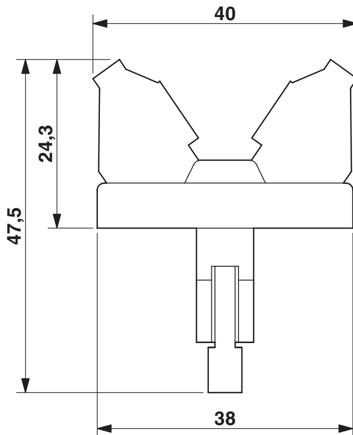
Rysunek wymiarowy
