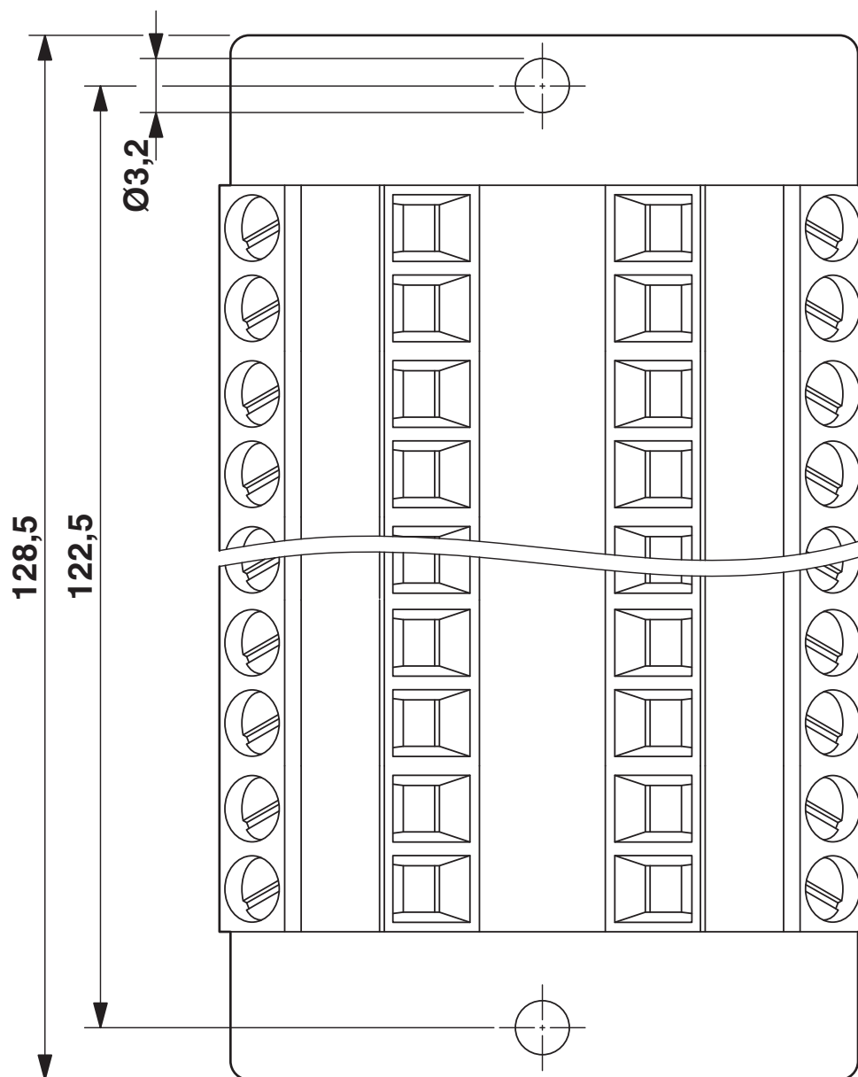
Rysunek wymiarowy
