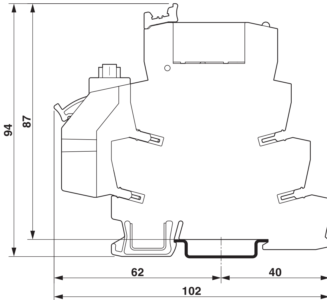
Rysunek wymiarowy
