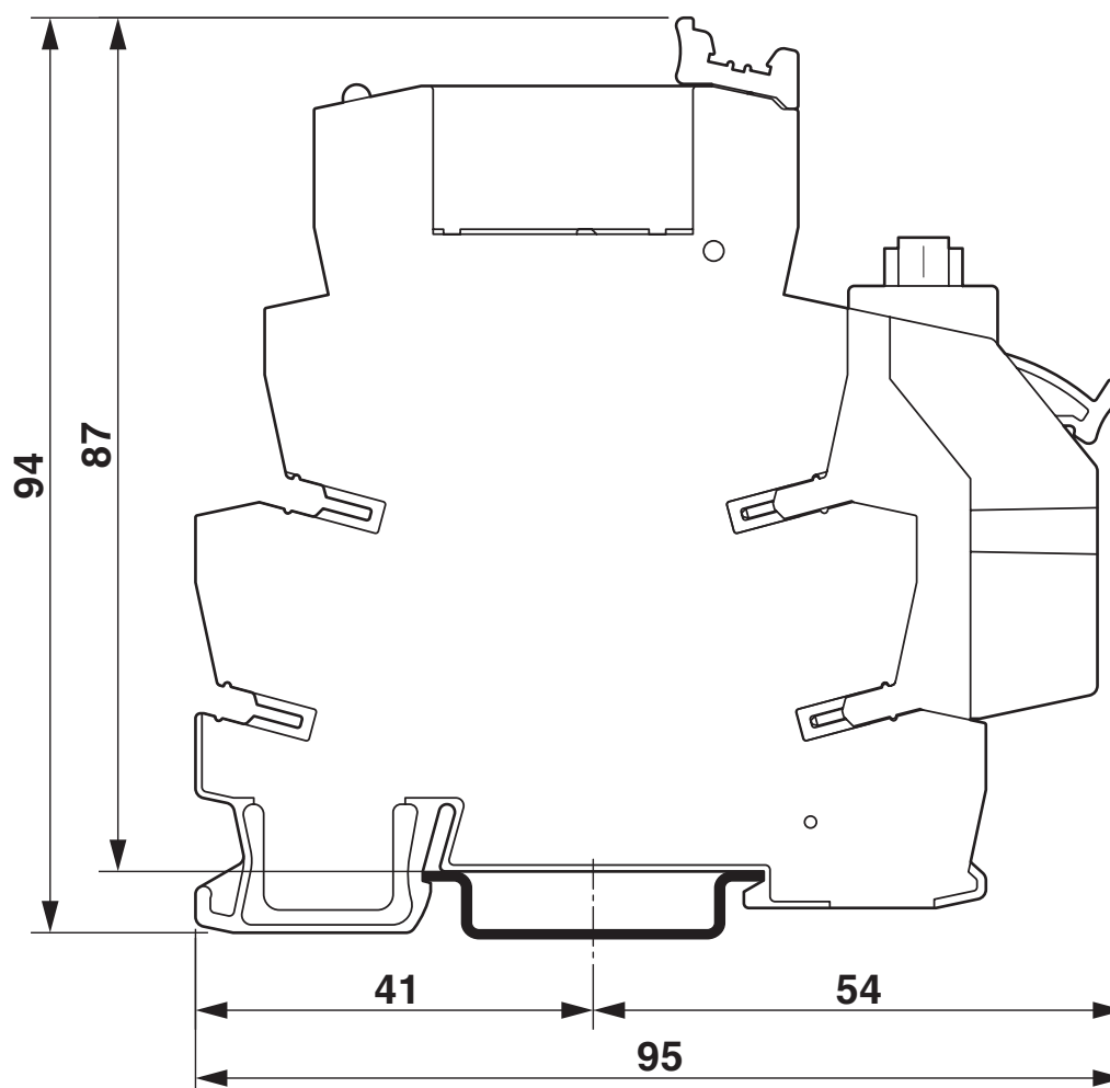
Rysunek wymiarowy
