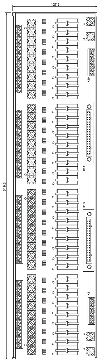
Rysunek wymiarowy
