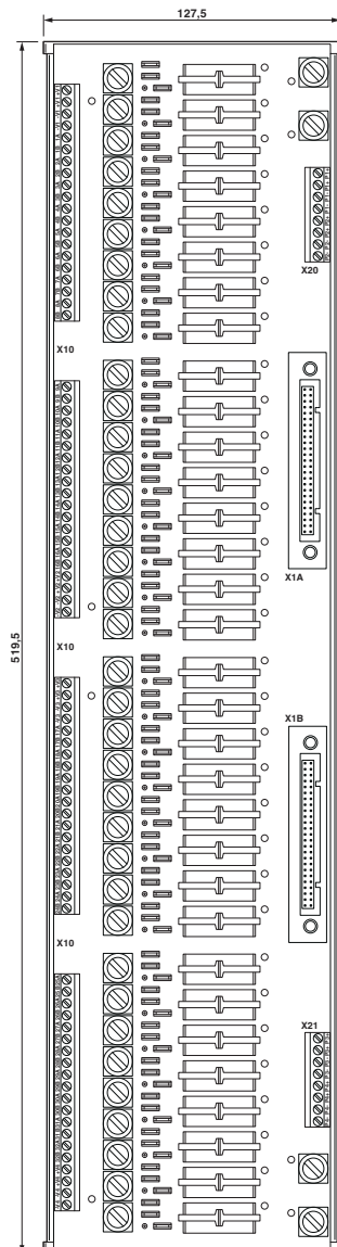
Rysunek wymiarowy
