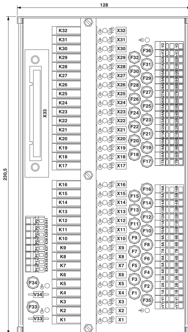
Rysunek wymiarowy
