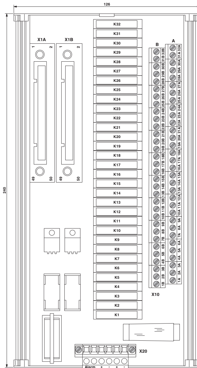
Rysunek wymiarowy
