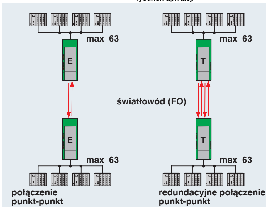
Połączenie punkt-punkt
