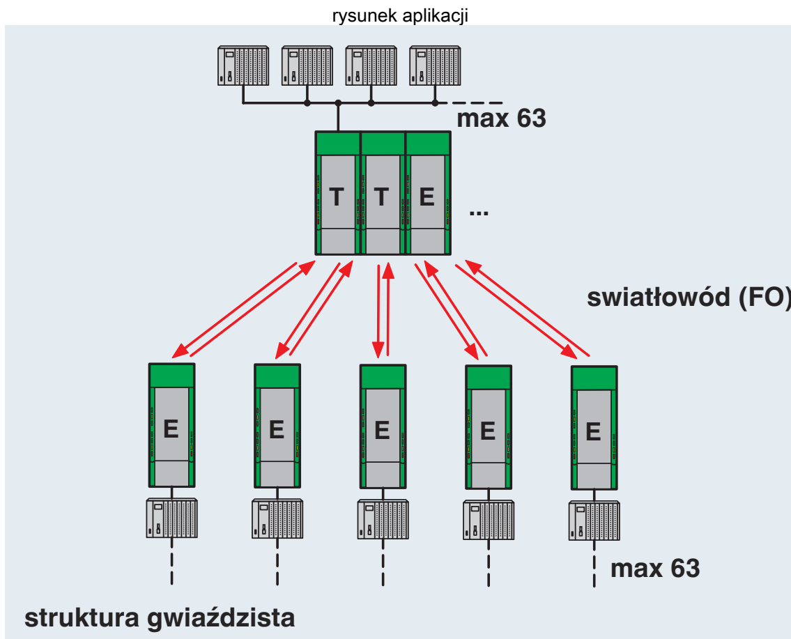
Struktura gwiazdowa
