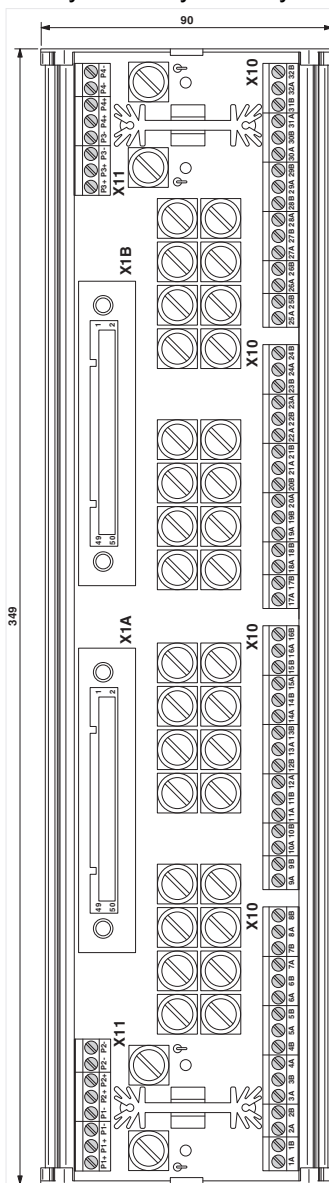
Rysunek wymiarowy
