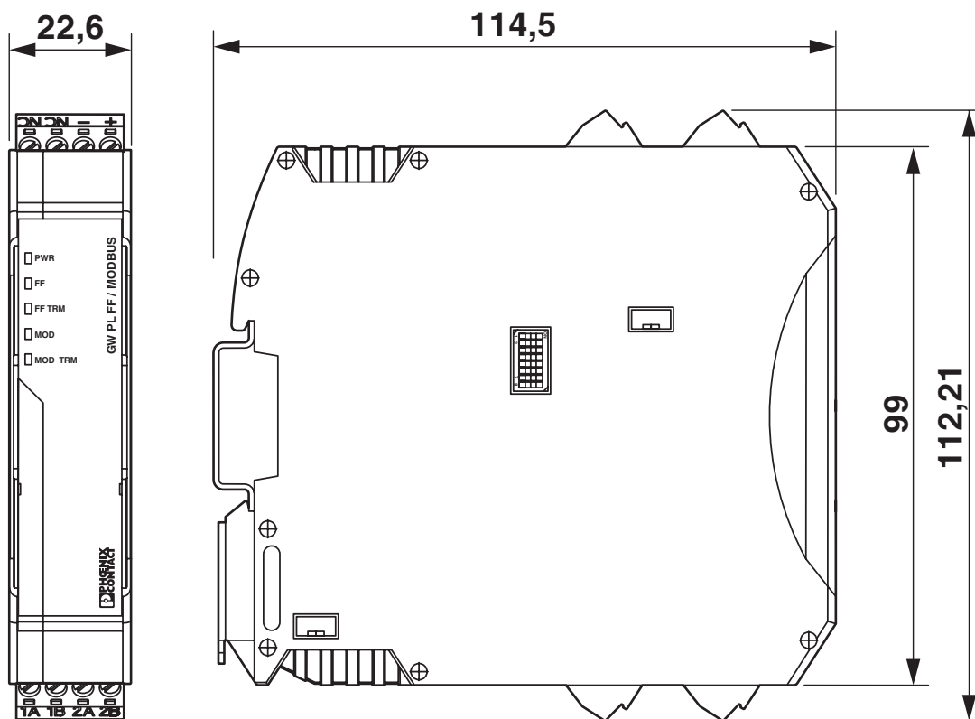
Rysunek wymiarowy
