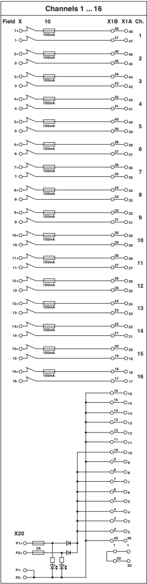
Schemat
