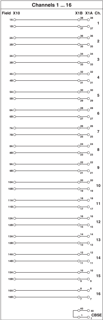
Schemat
