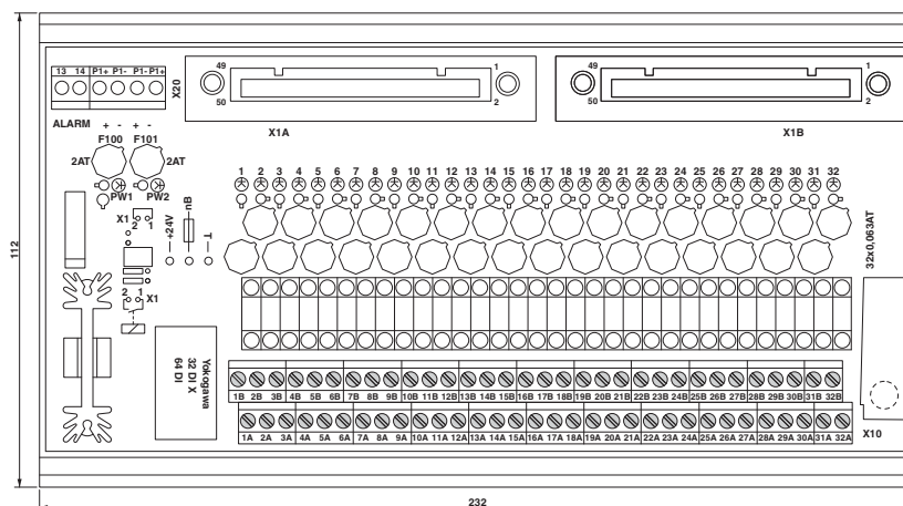
Rysunek wymiarowy
