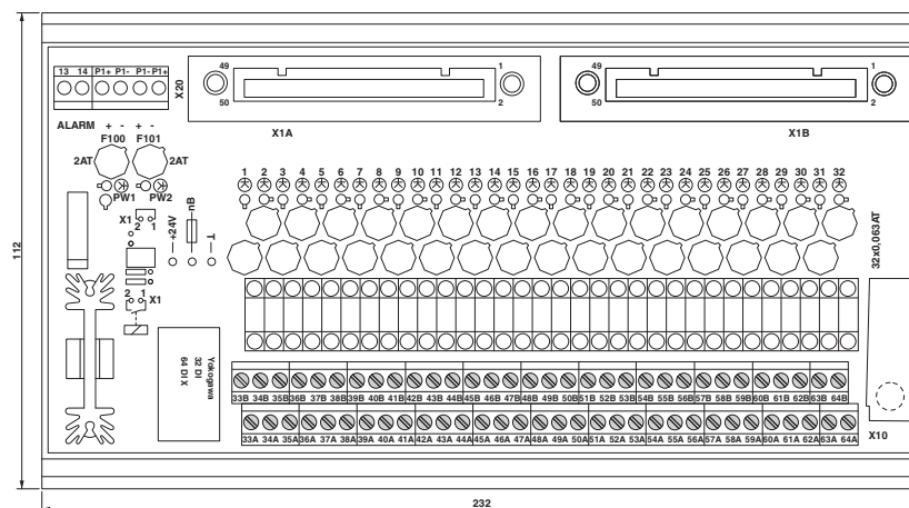
Rysunek wymiarowy
