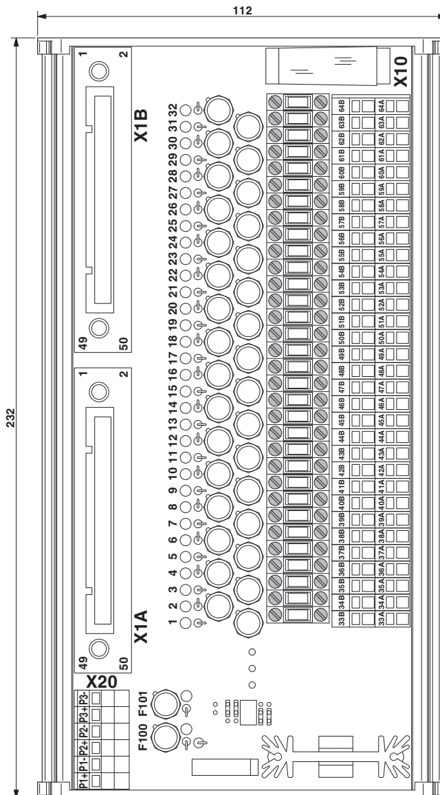
Rysunek wymiarowy
