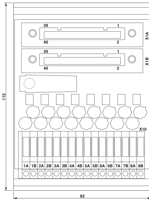
Rysunek wymiarowy
