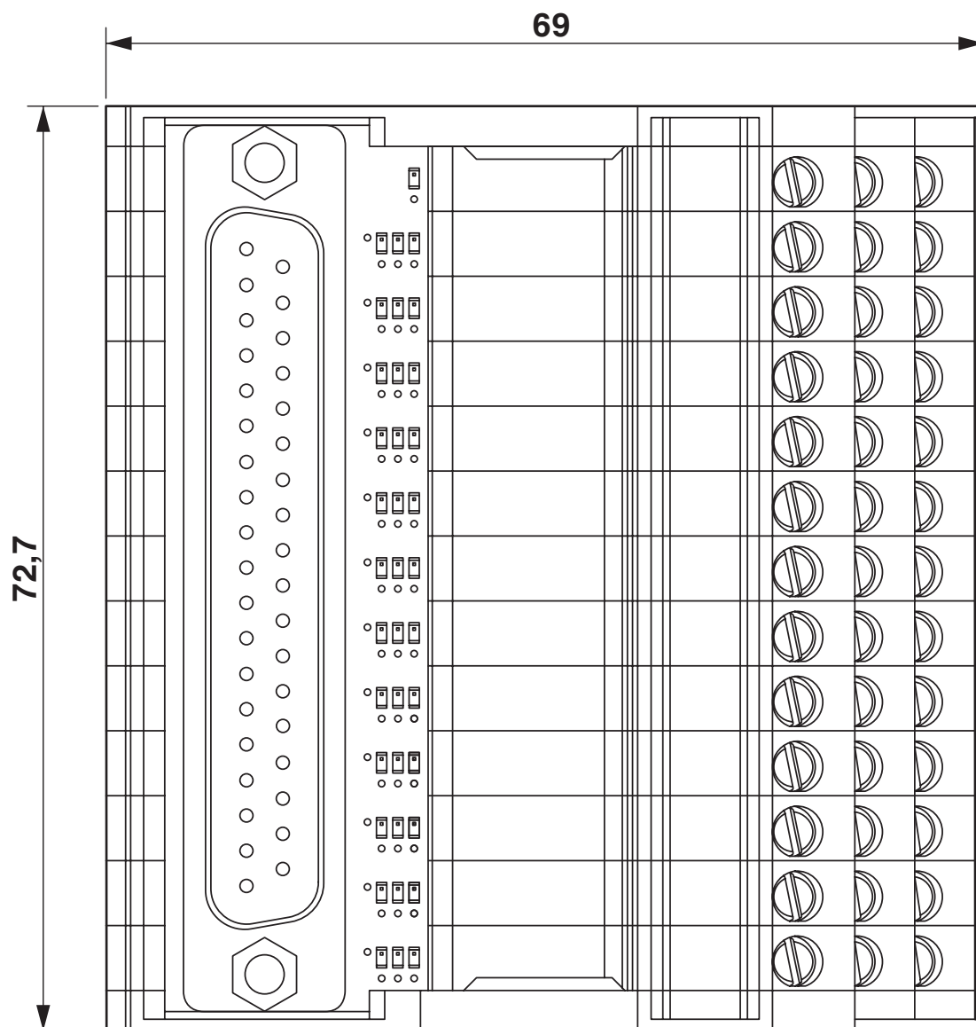
Rysunek wymiarowy
