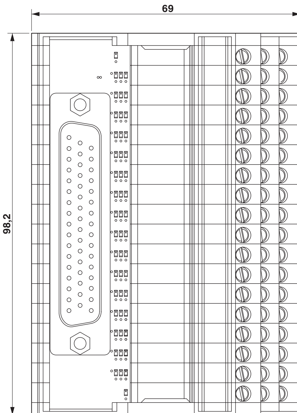
Rysunek wymiarowy
