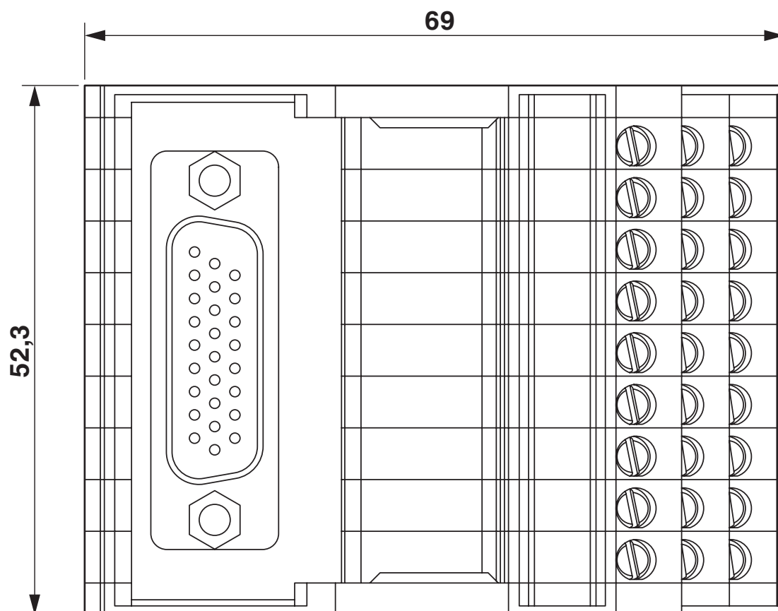
Rysunek wymiarowy
