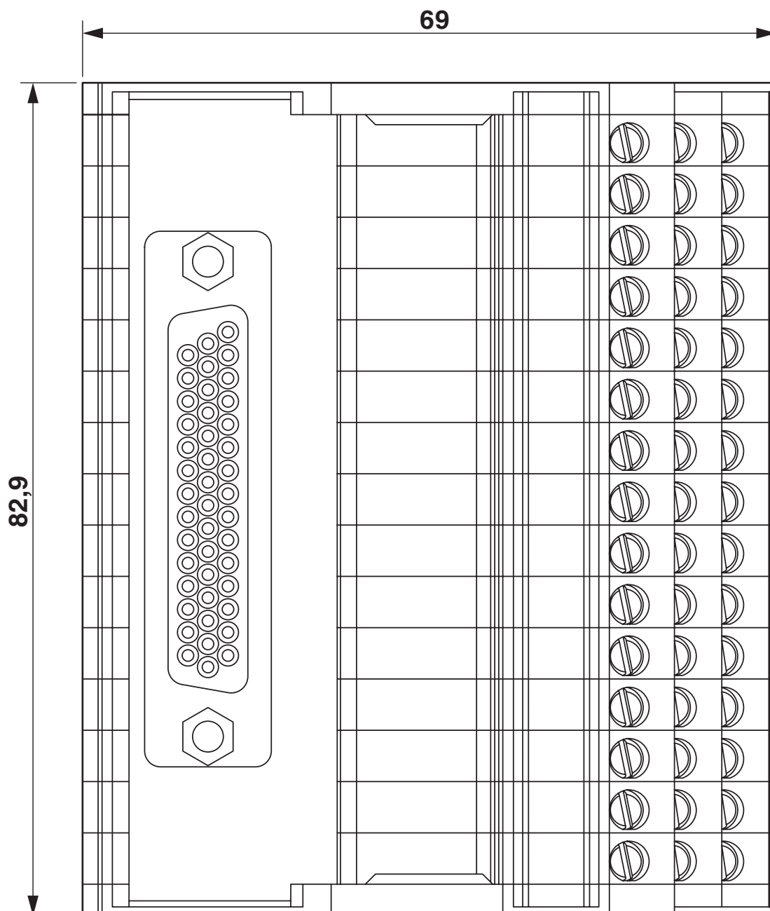
Rysunek wymiarowy
