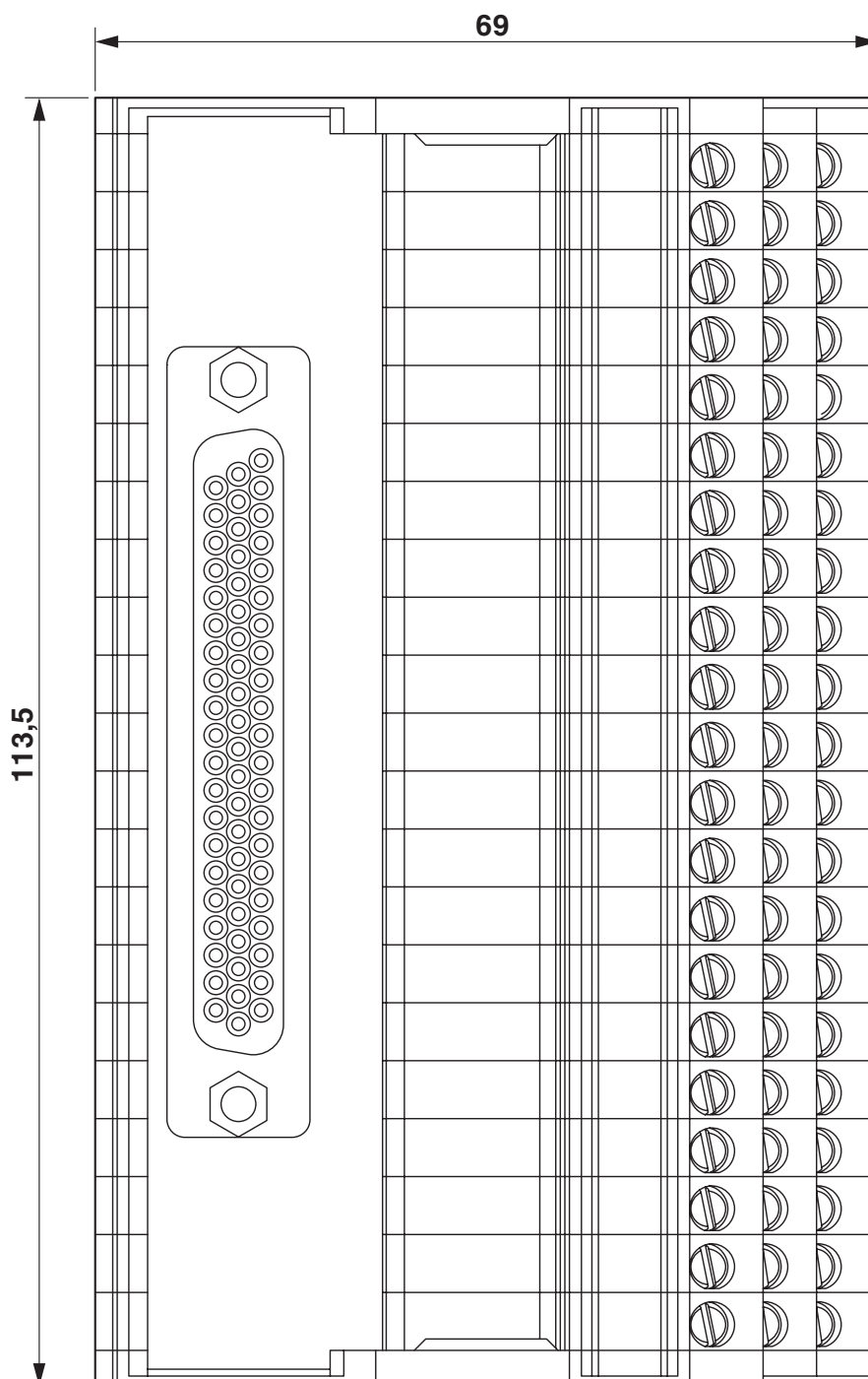
Rysunek wymiarowy
