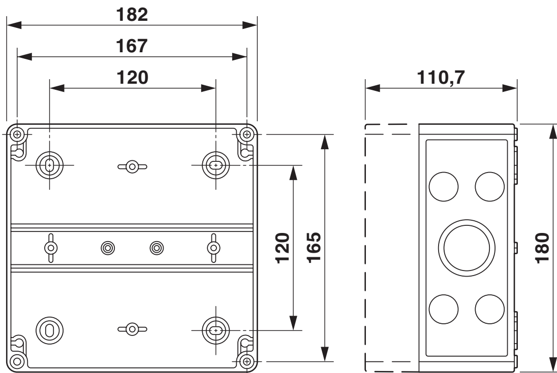
Rysunek wymiarowy
