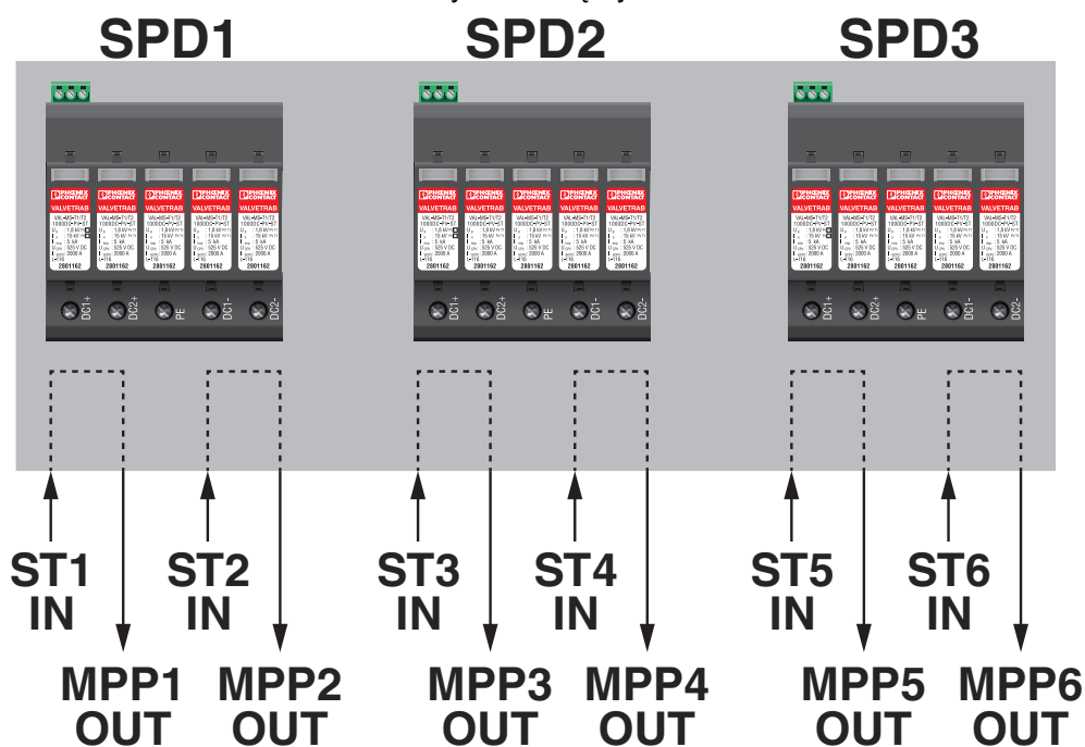
rysunek złączy
