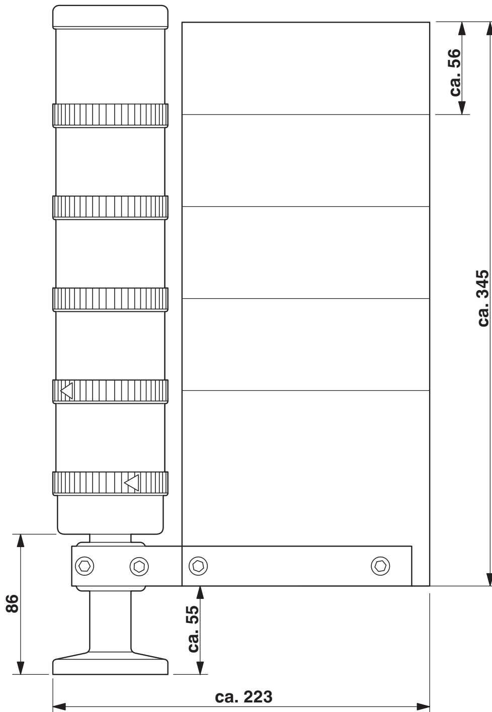
Rysunek wymiarowy
