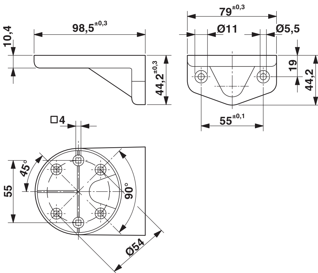
Rysunek wymiarowy
