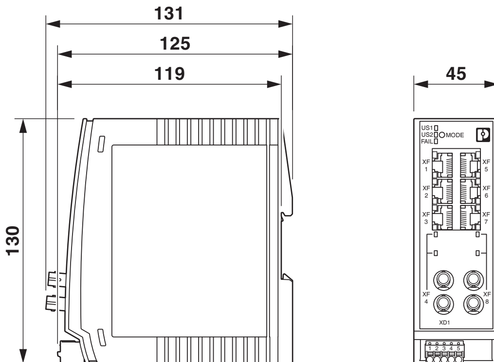
Rysunek wymiarowy
