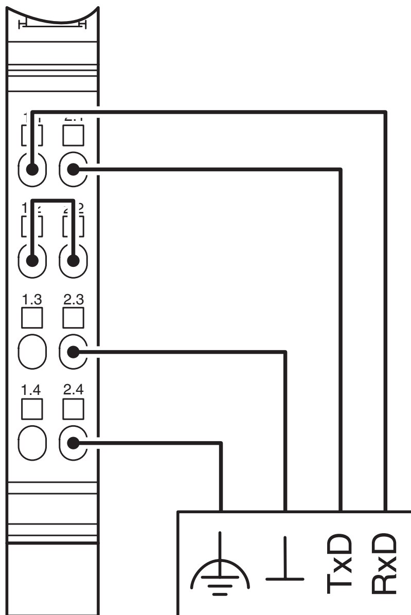
rysunek złączy
