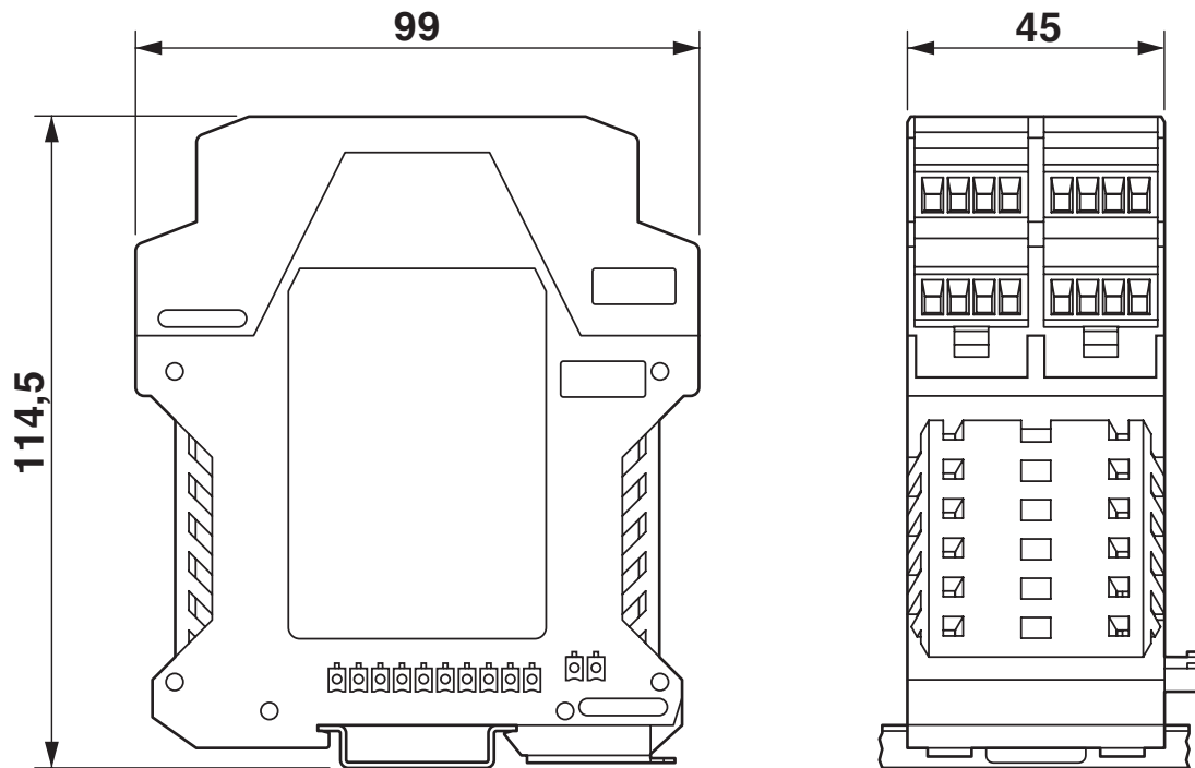
Rysunek wymiarowy
