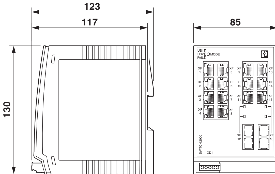
Rysunek wymiarowy
