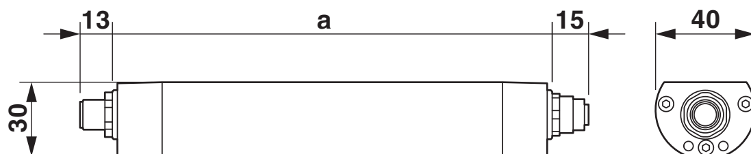
Rysunek wymiarowy
