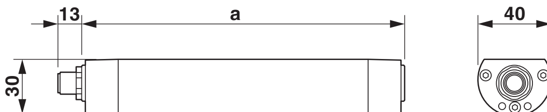
Rysunek wymiarowy
