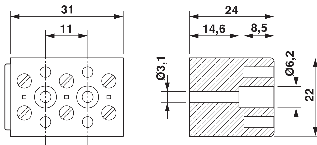
Rysunek wymiarowy
