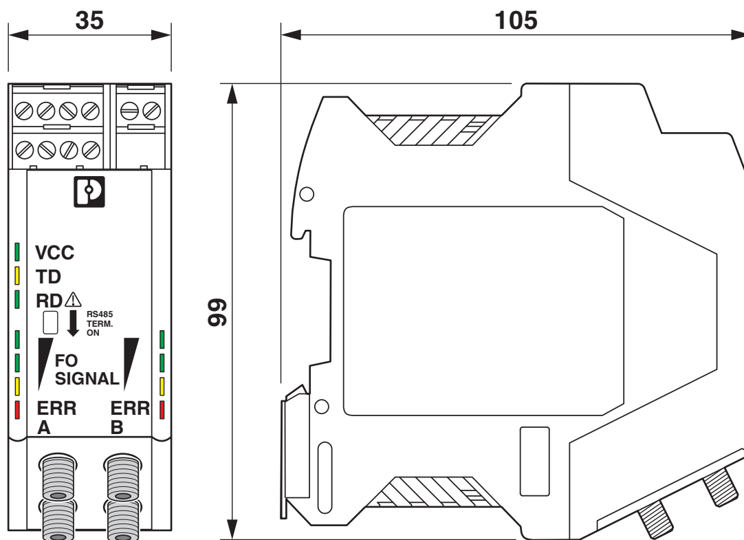
Rysunek wymiarowy
