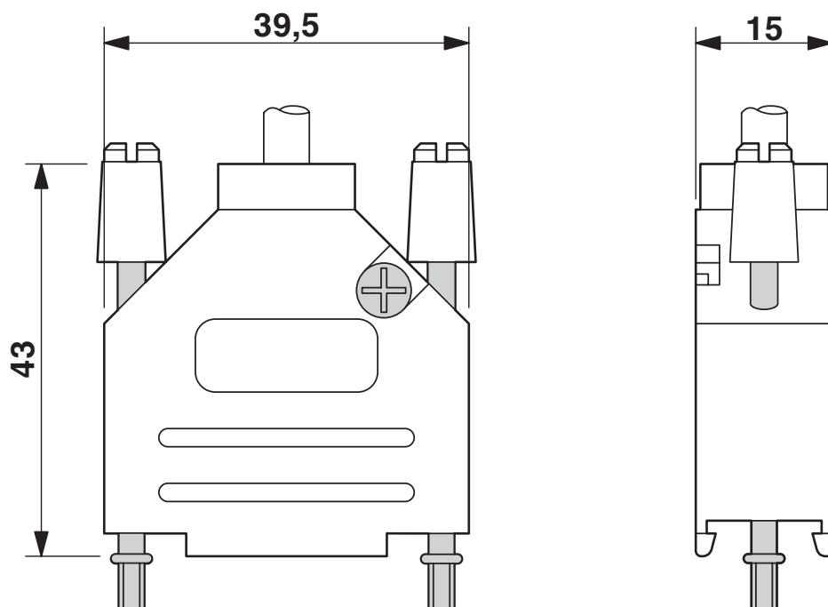
Rysunek wymiarowy
